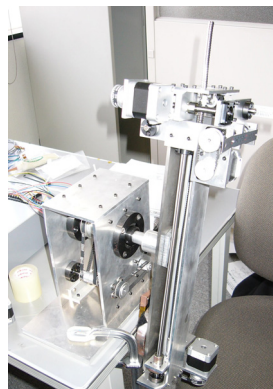
Morphable Beamの実験装置
